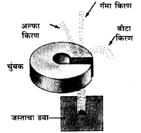
निरनिराळ्या प्रकारच्या किरणोत्सर्गावरील चुंबकाचा प्रभाव
